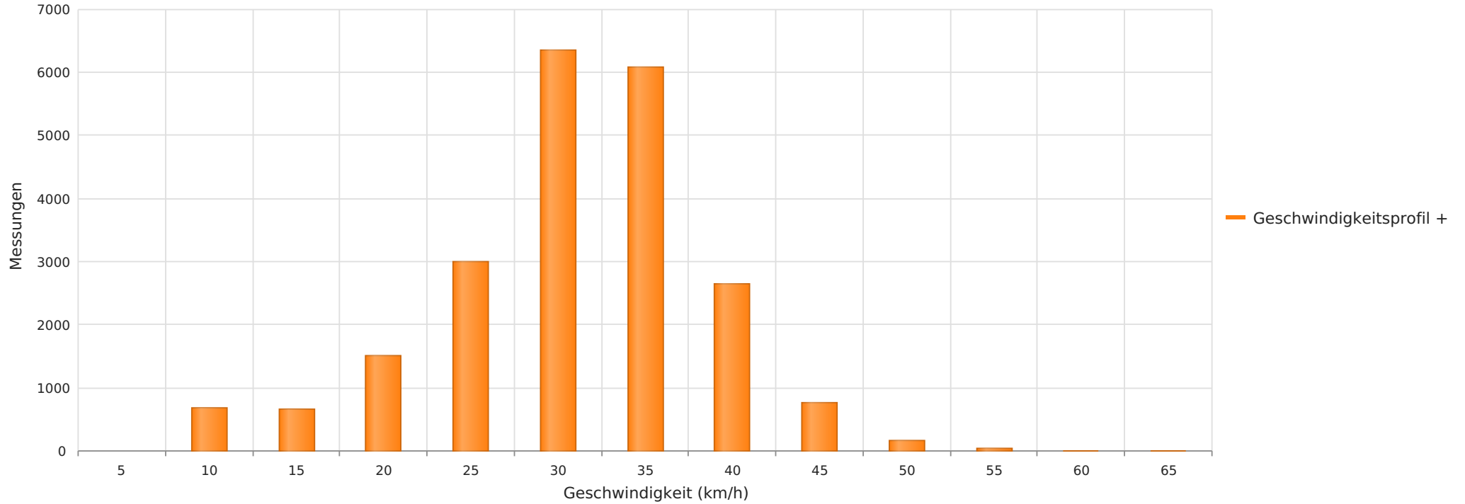
Lindenweg 18, Fahrtrichtung Selzerbachweg, 30 km/h Beschränkung Anzahl der Messwerte vs. Geschwindigkeit
