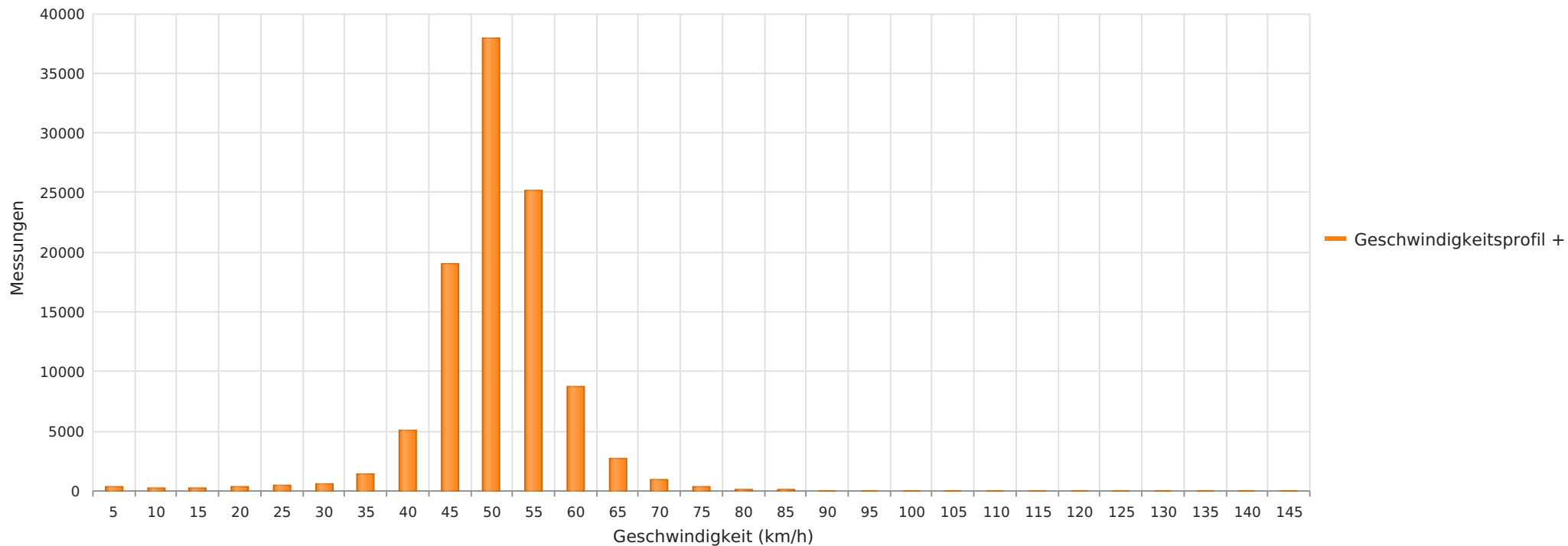
Rendeler Str. 87, Fahrtrichtung OA, 50 km/h Beschränkung Anzahl der Messwerte vs. Geschwindigkeit
