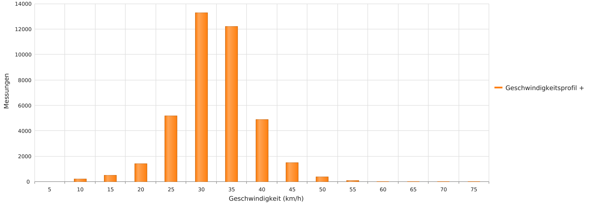
Hauptstraße, HsNr.32 , Fahrtrichtung OM, 30 km/h Beschränkung Anzahl der Messwerte vs. Geschwindigkeit
