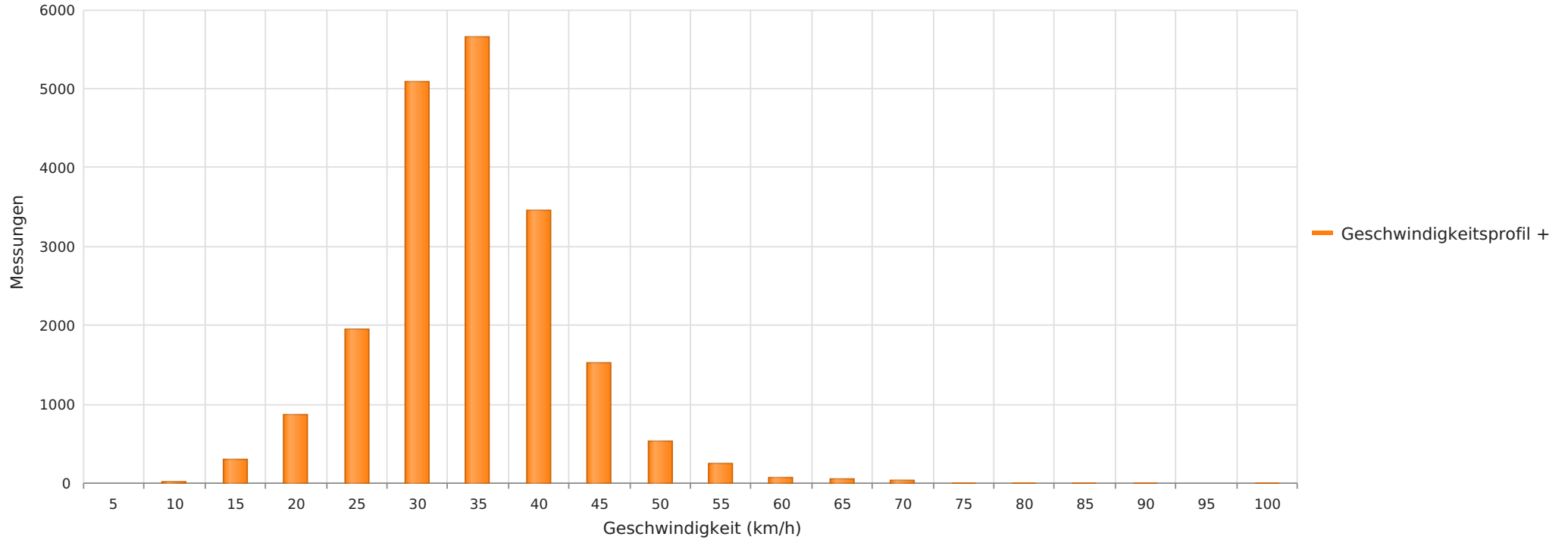
Dieselstr.Kiga, Fahrtrichtung BGZ Rathaus, 30 km/h Beschränkung Anzahl der Messwerte vs. Geschwindigkeit
